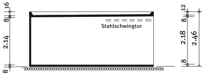
Schnitt
