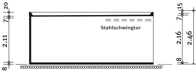
Schnitt
