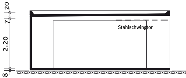
Schnitt
