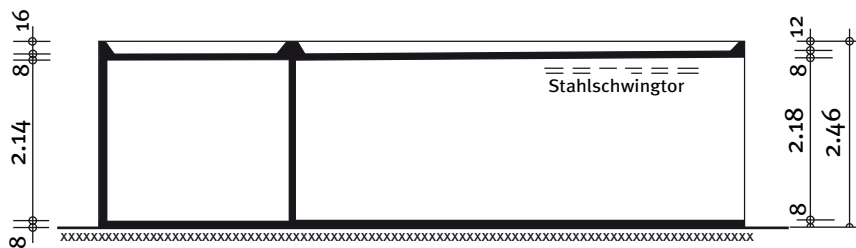
Schnitt
