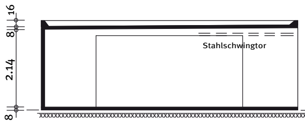
Schnitt
