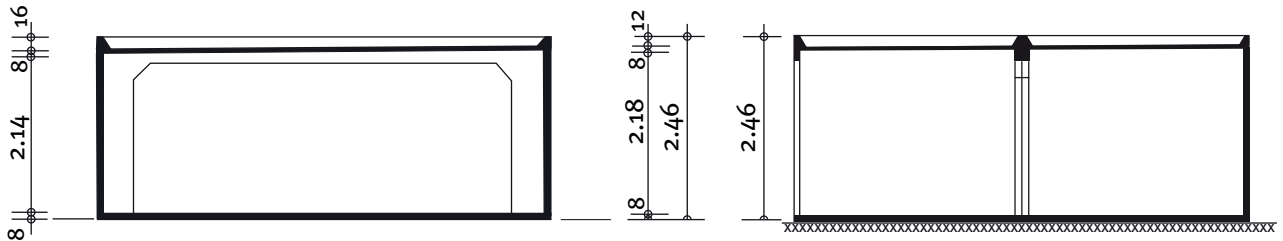
Querschnitt
