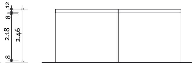
Rückansicht
