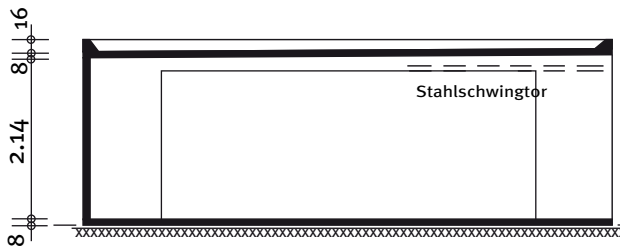
Schnitt
